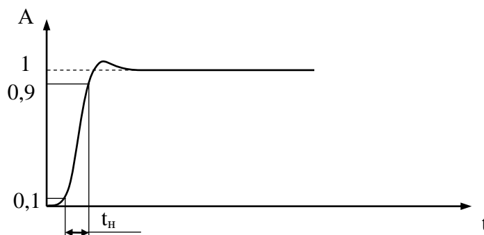
Рис. 5. Изображение испытательного импульса при измерении времени нарастания переходной характеристики t_H .
